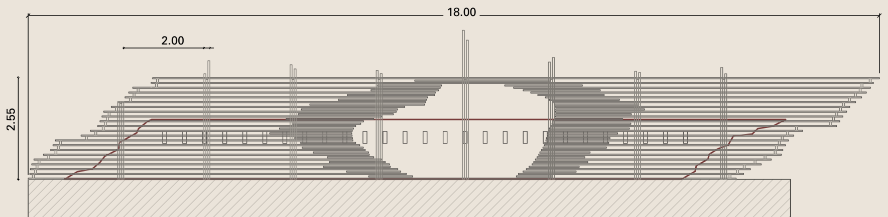
Aufriss gesamt
